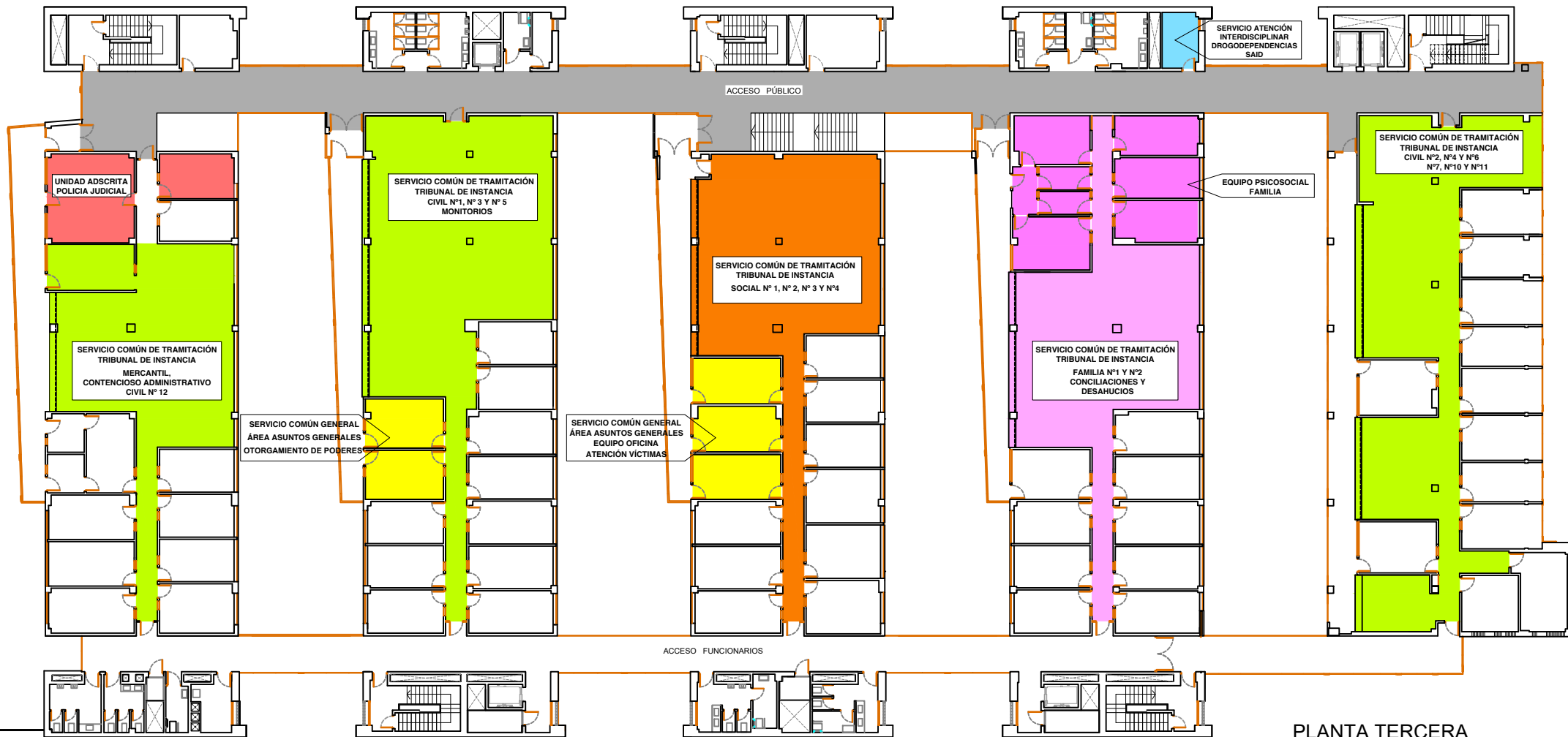
PLANTA TERCERA
